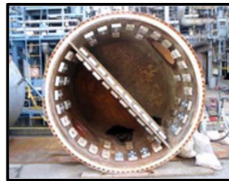
Sacrificial Anode
